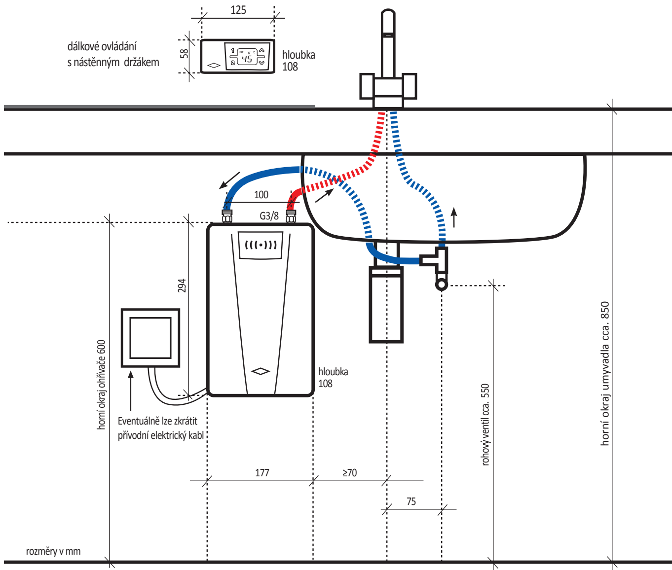
Příklad tlakové instalace
